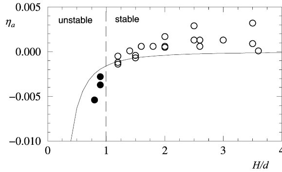
Fig. 4. Comparison of measurements (○ stable, ● unstable) and predictions (—) Eq. (6b) of the added damping for the plane jet. Fig. 4. Comparaison mesures (○ stable, ● instable) / prédictions (—), Éq. (6b) de l'amortissement ajouté pour le jet plan.
