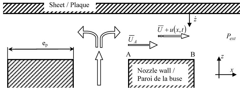
Fig. 5. Detailed sketch of the space between nozzle and sheet. Fig. 5. Schéma de détail de l'espace entre la buse et la plaque.
